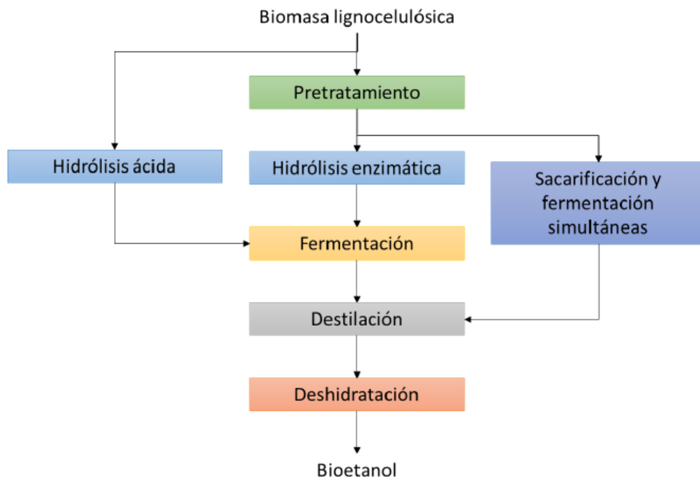
Imagen 6: Proceso de obtención de bioetanol
